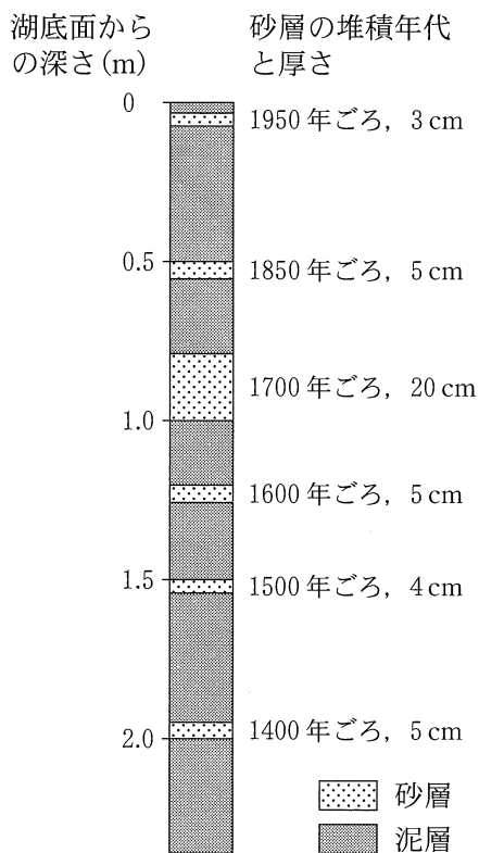
図 2 ある湖の底に堆積した完新世の地層の柱状図
