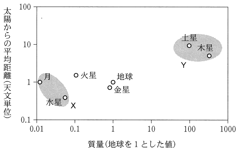
図 1 天体の質量と太陽からの平均距離
