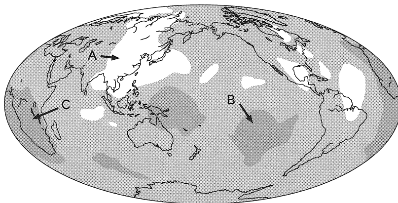
図 2 マンツル最下部(深さ約 2800 km)での P 波の地震波速度分布
