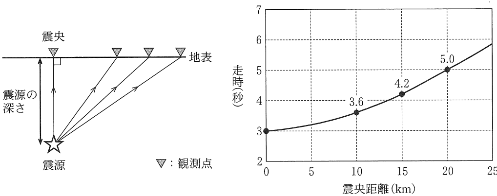
図 1 ある深さで発生した地震の P 波の伝わり方(左)とその走時曲線(右) 左図は波の伝わり方を模式的に示しており、縦横比は正確ではない。右図中の数字は、それぞれの震央距離での P 波の走時(秒)を表す。
